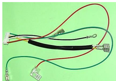
CABLEADO MODULO CAL. JUNKERS 8 T. (para CA452908) ORIGINAL 87044040410
