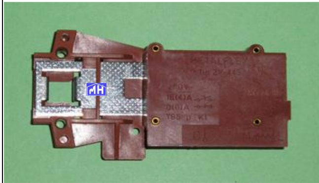
LA163604 - MICRO RETARDO LD BALAY SERIE T8201 AL 8217,5°GN.
