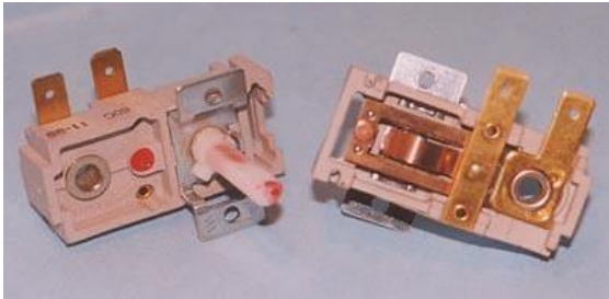
TERMOSTATO RADIADOR 40/100° EJE 20 mm.
