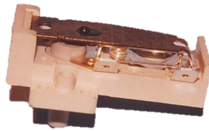
TERMOSTATO RADIADOR 5/45°
