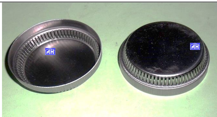
CC600401 - DIFUSOR QUEMADOR ORBEGOZO CHAPA N° 1 3,9 cm. CC600402 - DIFUSOR QUEMADOR ORBEGOZO CHAPA N° 2 5,8 cm. CC600403 - DIFUSOR QUEMADOR ORBEGOZO CHAPA N° 3 7 cm.
