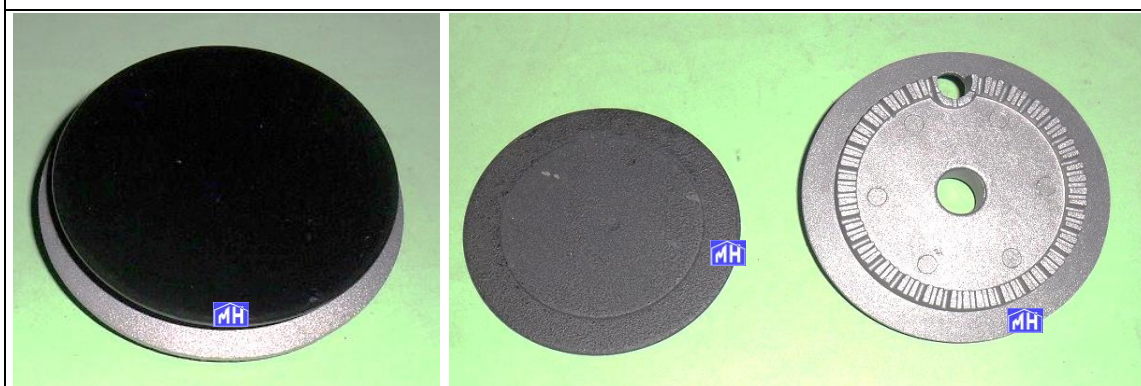
CC340411 - TAPETA QUEMADOR FAGOR/CORB./EDESA/ZAN. N° 1 5,5 cm. CC340412 - TAPETA QUEMADOR FAGOR/CORB./EDESA/ZAN. N° 2 7,2 cm. CC340413 - TAPETA QUEMADOR FAGOR/CORB./EDESA/ZAN. N° 3 10,2 cm. CC340507 - BASE QUEMADOR C/RANURA FAGOR/CORB./EDESA/ZAN. N° 1 3,7 cm. CC340508 - BASE QUEMADOR C/RANURA FAGOR/CORB./EDESA/ZAN. N° 2 5,2 cm. CC340509 - BASE QUEMADOR C/RANURA FAGOR/CORB./EDESA/ZAN. N° 3 8,3 cm.
