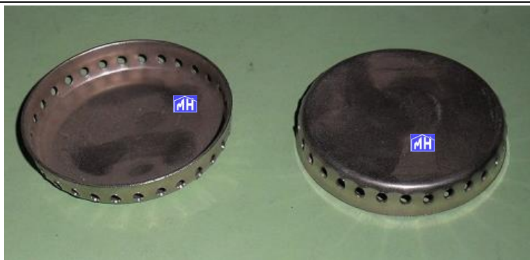
CC740401 - DIFUSOR QUEMADOR CORCHO CHAPA N° 1 3,5 cm. CC740402 - DIFUSOR QUEMADOR CORCHO CHAPA N° 2 5 cm. CC740403 - DIFUSOR QUEMADOR CORCHO CHAPA N° 3 6,5 cm.
