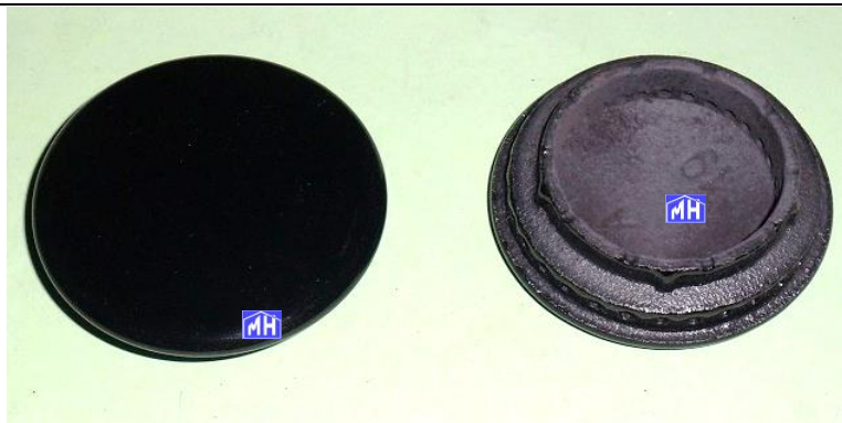
CC340407 - TAPETA QUEMADOR FAGOR FUNDICIÓN N° 1 3,7 cm. CC340408 - TAPETA QUEMADOR FAGOR FUNDICIÓN N° 2 5,6 cm. CC340409 - TAPETA QUEMADOR FAGOR FUNDICIÓN N° 3 7,2 cm. CC340410 - TAPETA QUEMADOR FAGOR FUNDICIÓN N° 4 7,7 cm.
